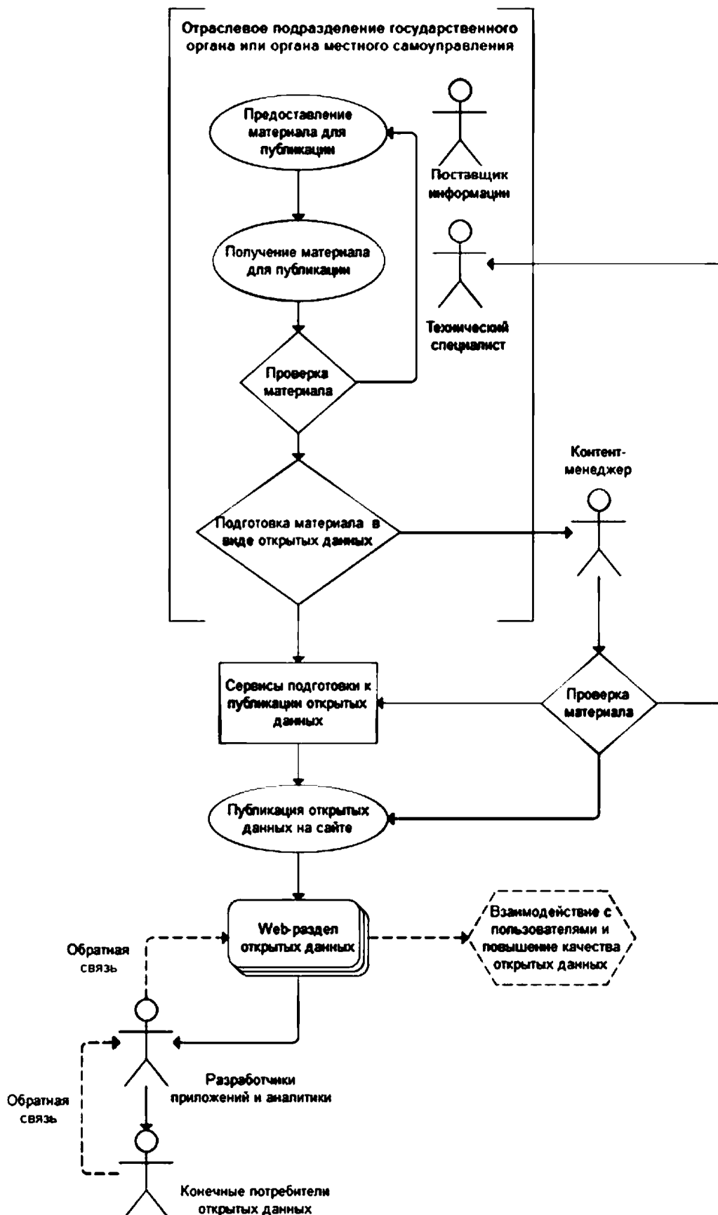
Рисунок 1 – Схема взаимодействия при публикации набора открытых данных
